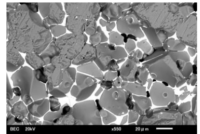
Fig. 1 \text{ZnO}-x \text{ mol}\% \text{ Bi}_2\text{O}_3 の粒子と粒界相
