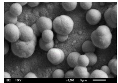
Fig. 1 \text{ZnO}-x \text{ mol}\% \text{ Bi}_2\text{O}_3 の粒子と粒界相
